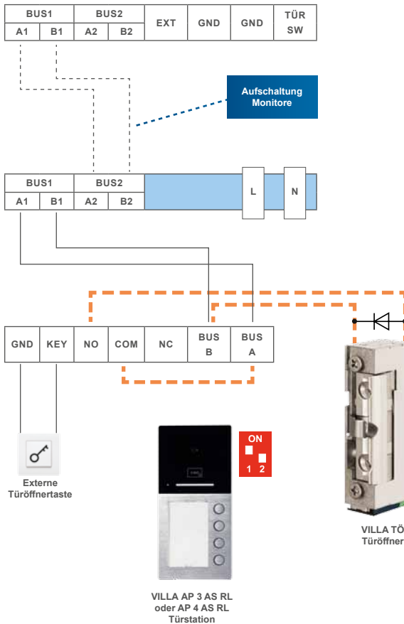
VILLA NG Netzgerät
