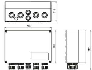
Maßbild DCU 2 YPV 1100 2M 2S
